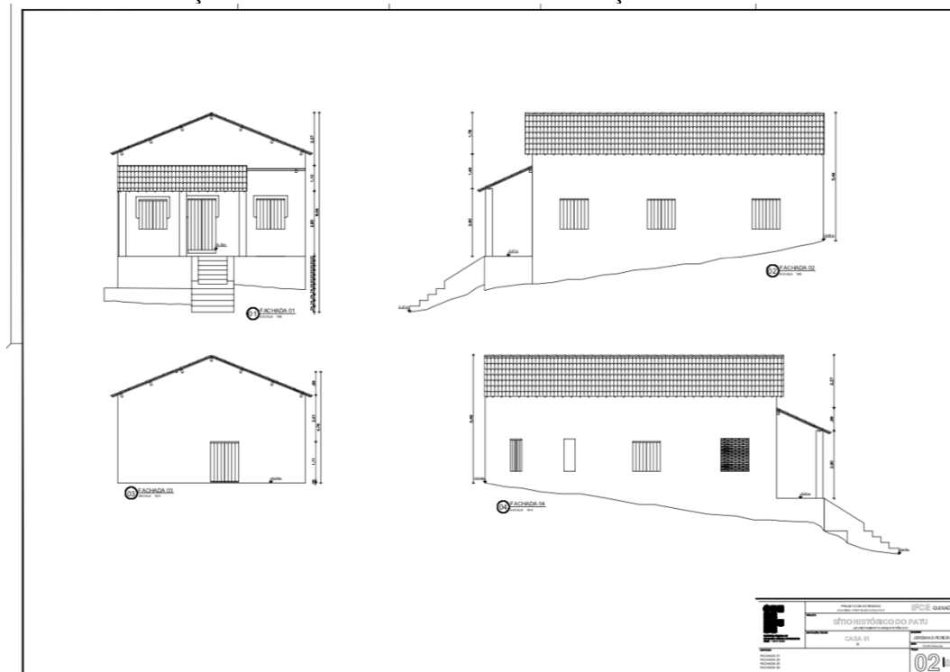
Ilustração 8 – Desenho técnico de uma das edificações do Sítio Histórico.
