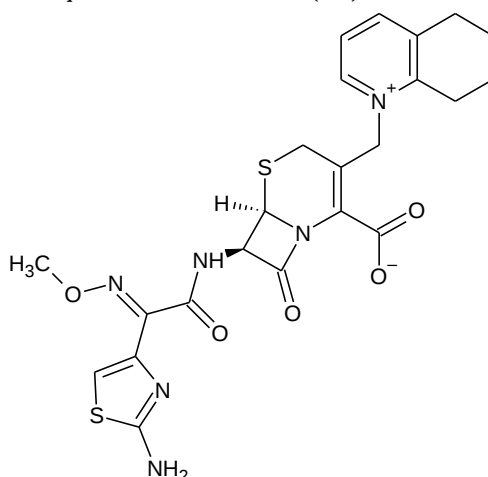
Figura 5: Estrutura química bidimensional (2D) do antibiótico Cefquinoma
