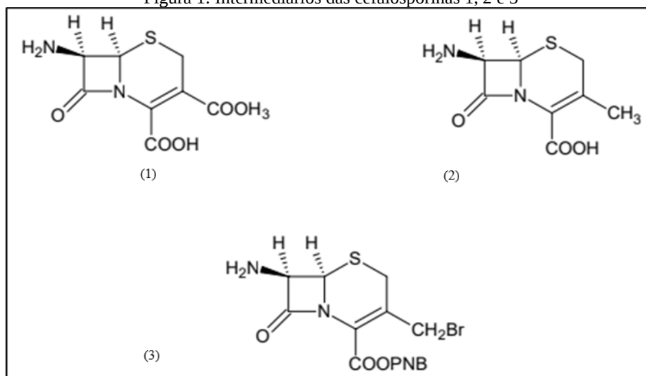
Figura 1: Intermediários das cefalosporinas 1, 2 e 3
