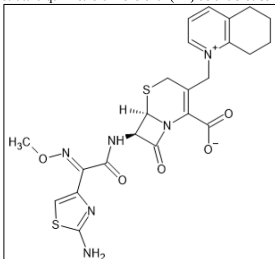
Figura 3: Estrutura química bidimensional (2D) do antibiótico Cefquinoma
