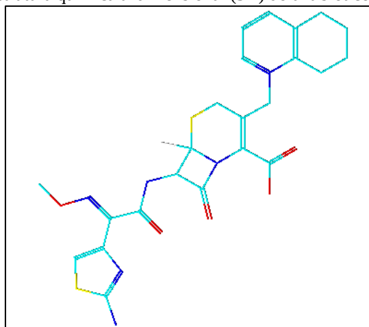
Figura 6: Estrutura química tridimensional (3D) do antibiótico Cefquinoma
