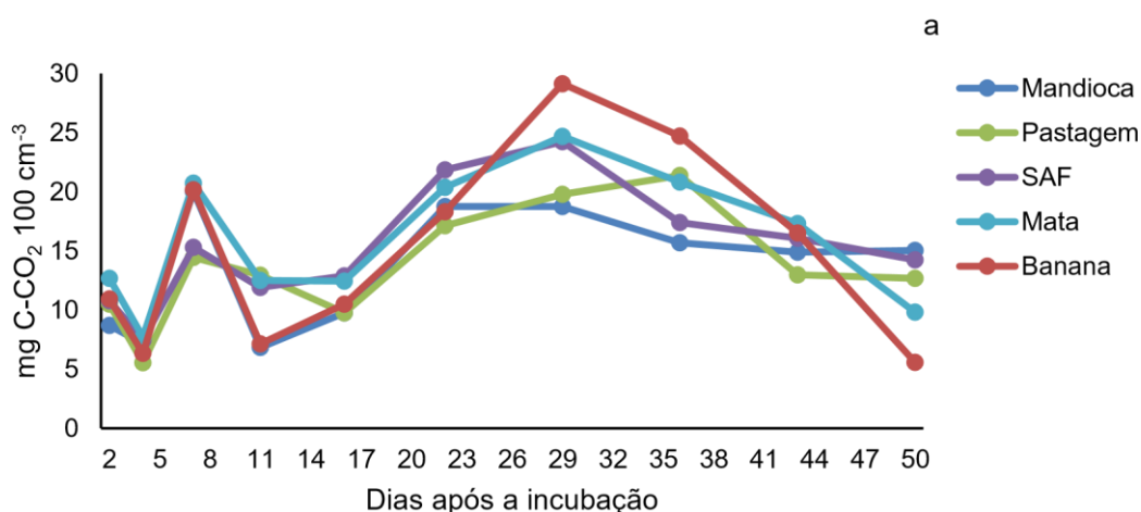
Figura 1. Evolução de C-CO 2 nas amostras (0-20cm) incubadas até os 50 dias nos meses de abril (a), junho (b) e agosto (c).
