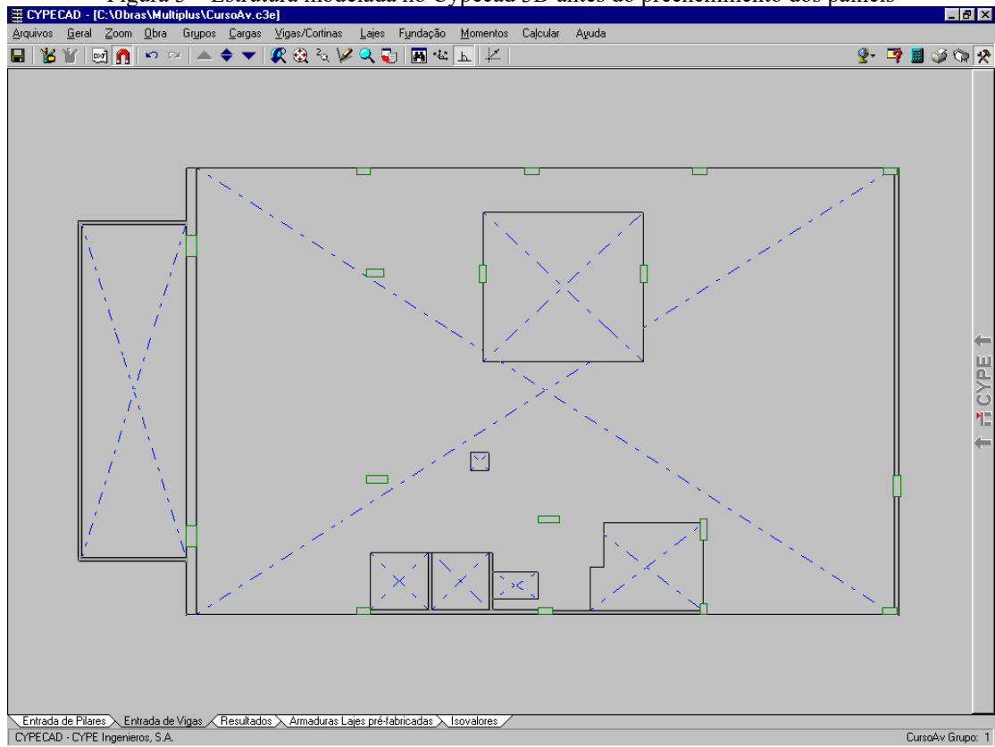
Figura 3 – Estrutura modelada no Cypecad 3D antes do preenchimento dos painéis
