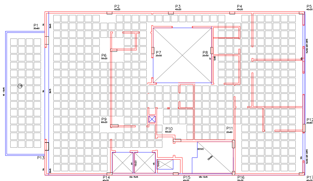
Figura 2 – Planta de Formas / Locação das alvenarias
