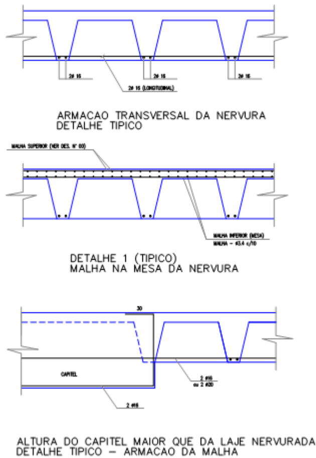
Figura 7 – Detalhamento das armaduras das nervuras
