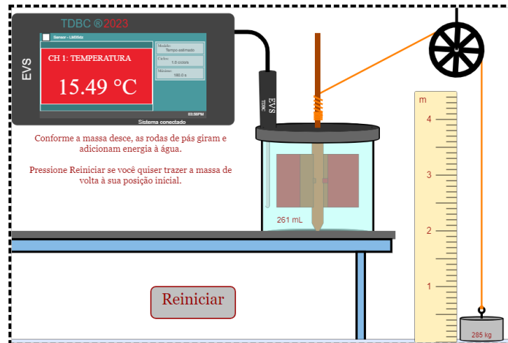
Figura 05: Momento de chegada do tracionador ao solo com dados a serem coletados pelo estudante.
