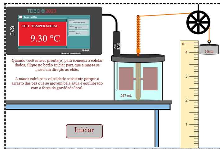
Figura 02: EVS – Equivalente Termomecânico
