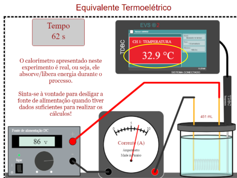
Figura 12: Destaque da temperatura da água doce após cerca de 60 segundos de aquecimento.
