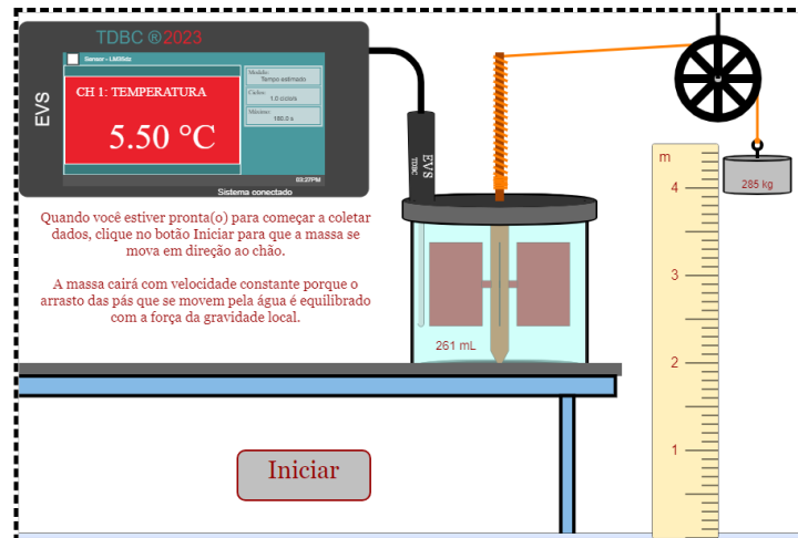
Figura 04: Momento inicial do EVS – Equivalente Termomecânico EVS - Equivalente Termomecânico
