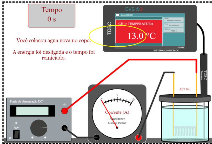
Figura 10: Destaque na temperatura aferida pelo TDBC.
