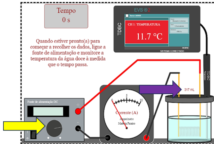
Figura 07: Tela inicial do EVS – Equivalente Termoeletrico. Equivalente Termoeletrico
