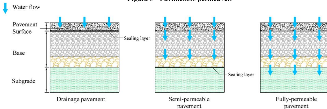
Figura 3 - Pavimentos permeáveis
