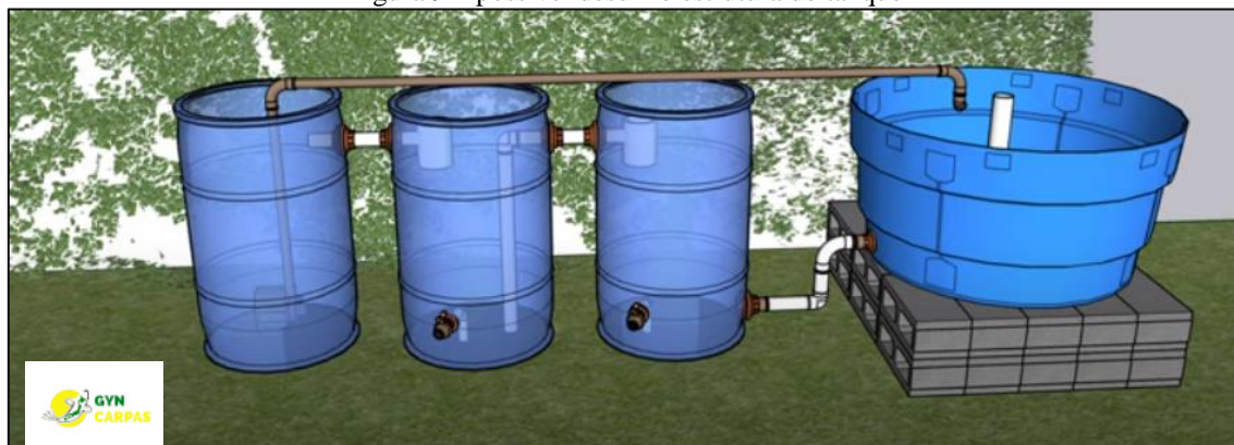
Figura 9 – possível desenho estrutura do tanque
